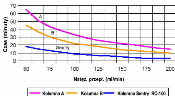
Czas odpowiedzi od natężenie przepływu
