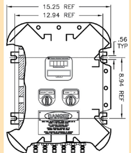
2020 Depth=11[279.4]
